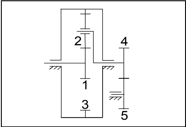
Схема зубчатого механизма
